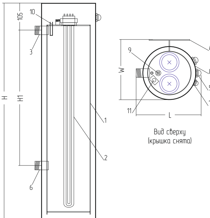
Вид сверху (крышка снята)
